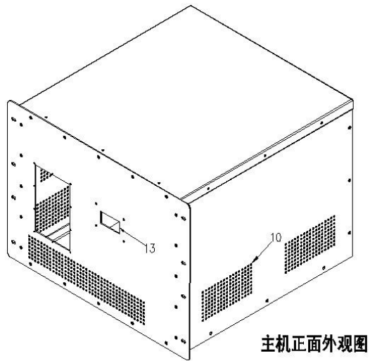
图 2.9 主机正面外观图
