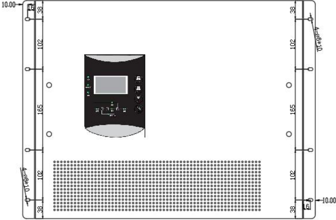
图 2.4 15KVA 机器面板尺寸图
