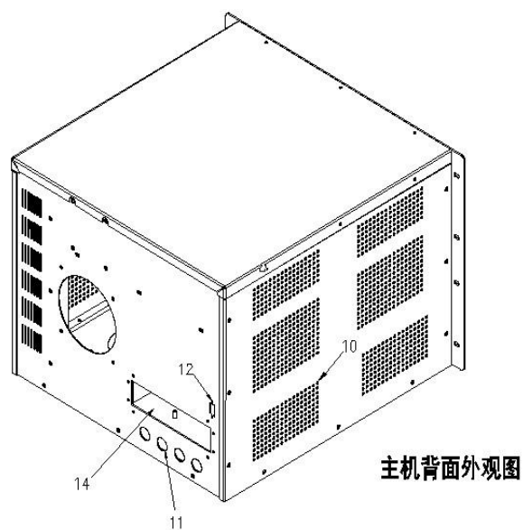
图 2.10 主机背面外观图
