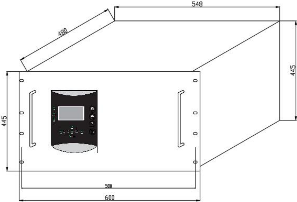
图 2.3 15KVA 机器尺寸（宽 600*深 480*高 445mm）
