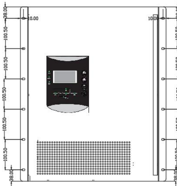
图 2.4 8-10KVA 实物面板图（电力逆变电源 UPS 面板图）
