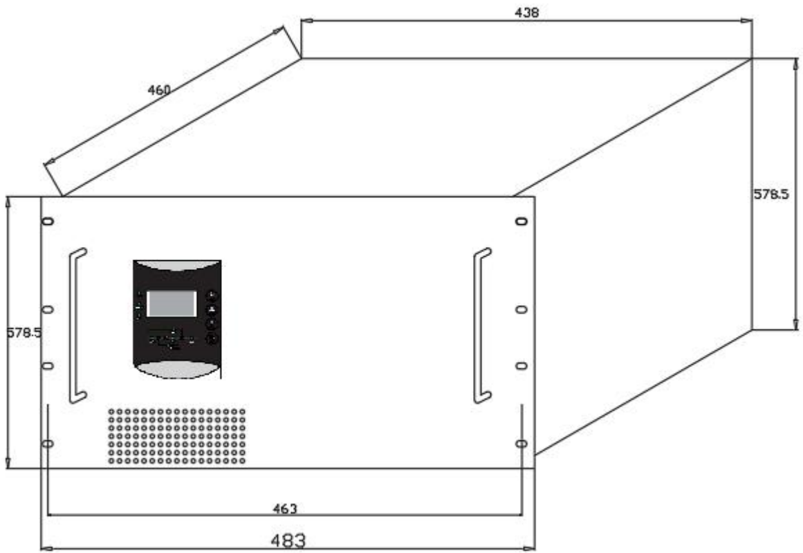
图 2.3 8-10KVA 机器尺寸（宽 483*深 460*高 578.5mm）
