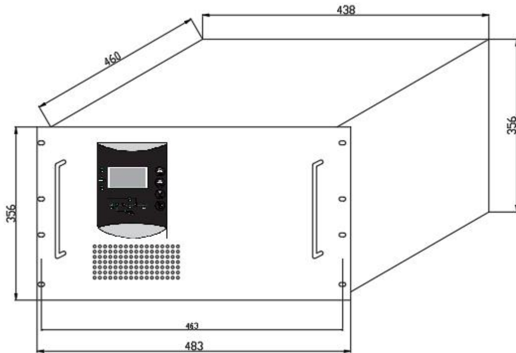
图 2.1 5KVA 机器尺寸（宽 483*深 460*高 356mm）
