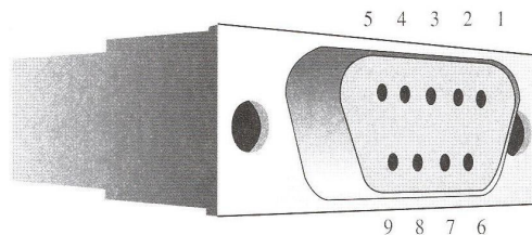
图 7.2 DB9 接脚信号
