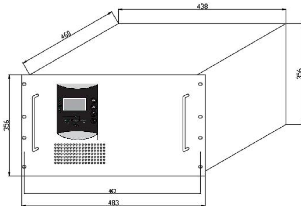
图 3.3 3-6KVA 机器尺寸（宽 483*深 460*高 356mm）
