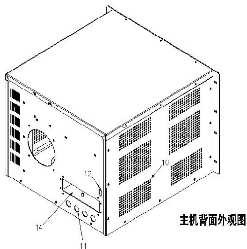
图 2.10 主机背面外观图
