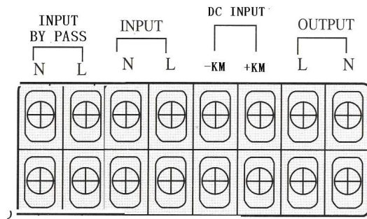
图 2.7 接线排接线图
