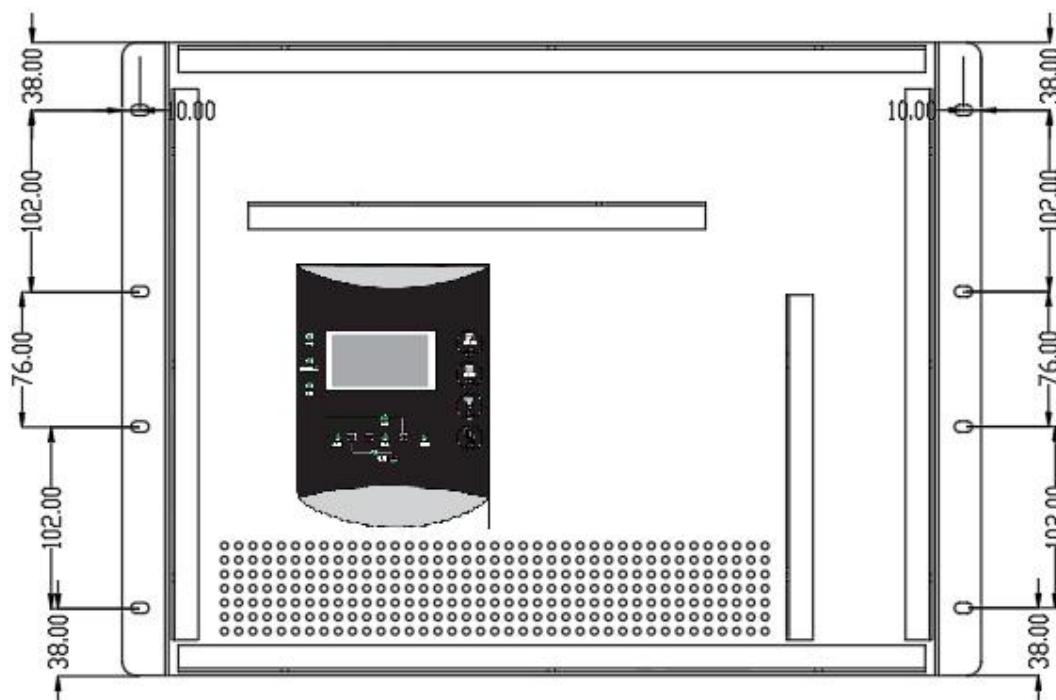
图 3.4 3-6KVA 实物面板图（电力逆变电源 UPS 面板图）
