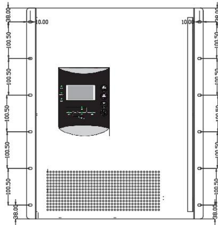
图 3.5 8-10KVA 机器尺寸 (宽 483*深 460*高 578.5mm)
