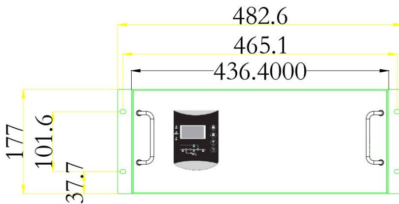
图 3.2 3KVA 实物面板图（电力逆变电源 UPS 面板图）
