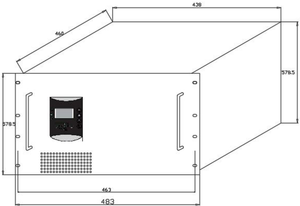
图 3.5 8-10KVA 机器尺寸 (宽 483*深 460*高 578.5mm)
