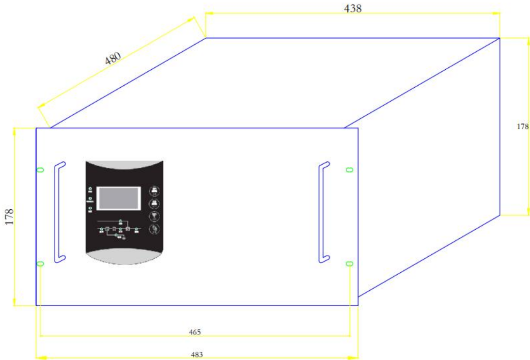
图 3.1 3KVA 机器尺寸（宽 483*深 460（不含把手）*高 178mm）
